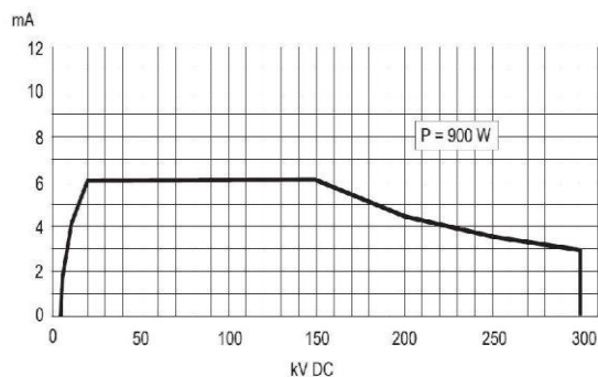
Charakterystyka mocy
